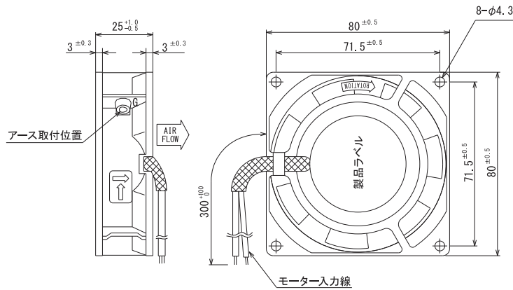
外形图
